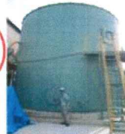
廃棄うどんからメタンガスを作る直径8メートルのタンク。発電設備と直結し、24時間の発電が可能という=高松市香南町西庄(朝日新聞デジタル)
